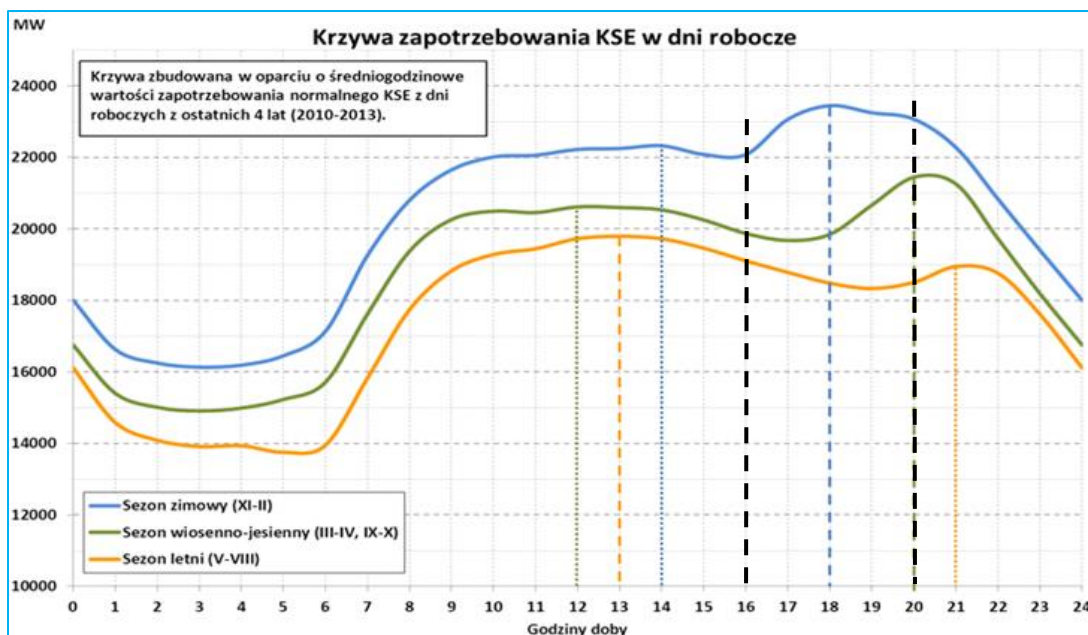
Rysunek 23 Dobowy rozkład zapotrzebowania mocy Krajowej Sieci Energetycznej w okresie roku [Źródło: PSE]
