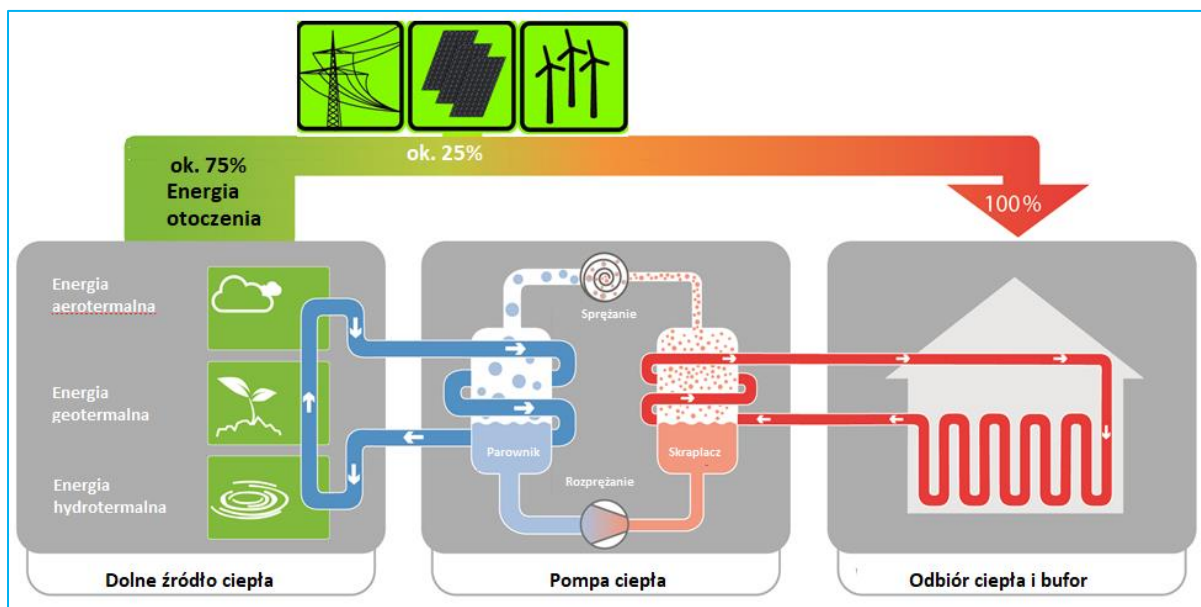
Rysunek 19 Pompy ciepła są gotowe na pełną dekarbonizację ciepła i w perspektywie najbliższych dziesięcioleci mogą produkować ciepła będące 100% OZE, bez żadnej emisji pyłów zawieszonych [Źródło: BWP/PORT PC]
