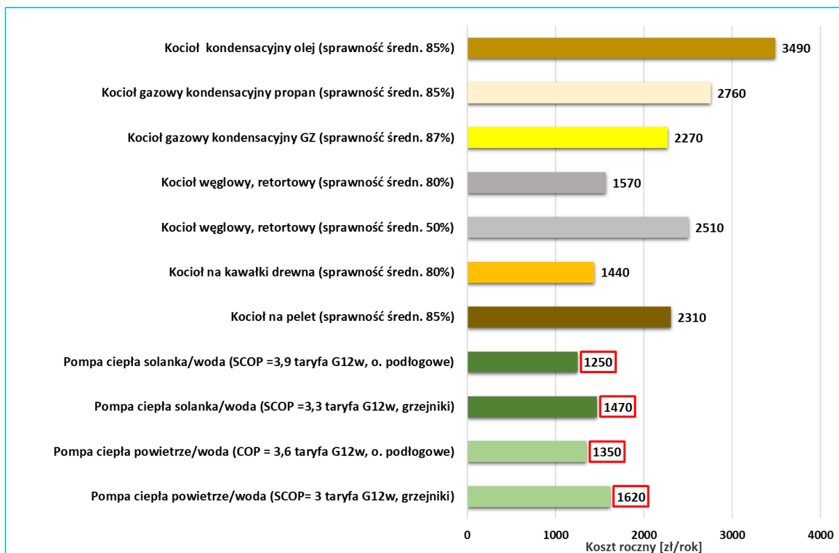
Rysunek 5 Roczny koszt ogrzewania budynku o pow. 130 m 2 wg WT 2021, wraz przygotowaniem c.w.u. (4 os. po 50 l/dobę) - dane styczeń 2018
