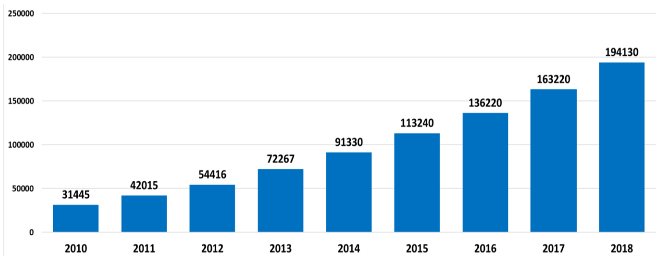
Rysunek 3 Zakumulowana, łączna liczba pracujących w Polsce pomp ciepła do centralnego ogrzewania i c.w.u. (sztuk)
